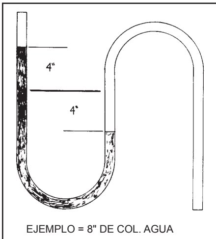
ILUSTRACIÓN #8 MEDICIÓN DE LA COLUMNA DE AGUA
