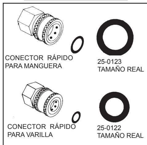
ILUSTRACIÓN #16 ACOPLADORES RÁPIDOS
