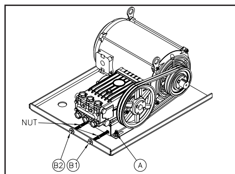
ILUSTRACIÓN #18 AJUSTE DE TENSIÓN DE CORREA
