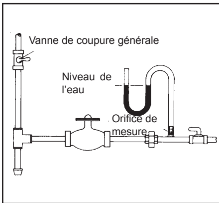
SCHÉMA N° 7 FABRICATION D'UN MANOMÈTRE
