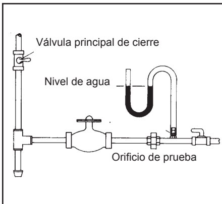
ILUSTRACIÓN #8 MEDICIÓN DE LA COLUMNA DE AGUA
