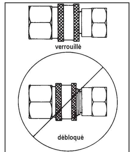
SCHÉMA N° 6 RACCORD RAPIDE
